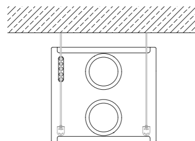
Подвесной монтаж
