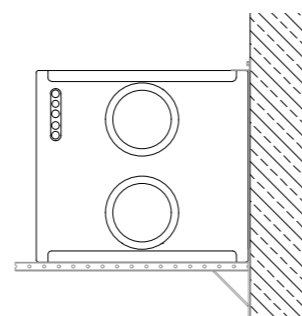
Настенный монтаж
